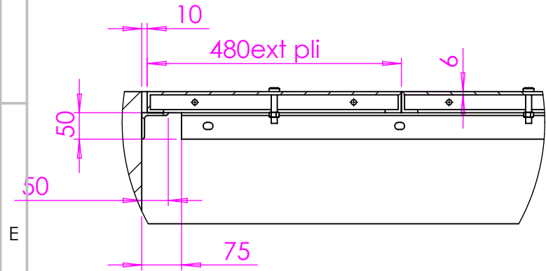
DÉTAIL B ECHELLE 1 / 10
