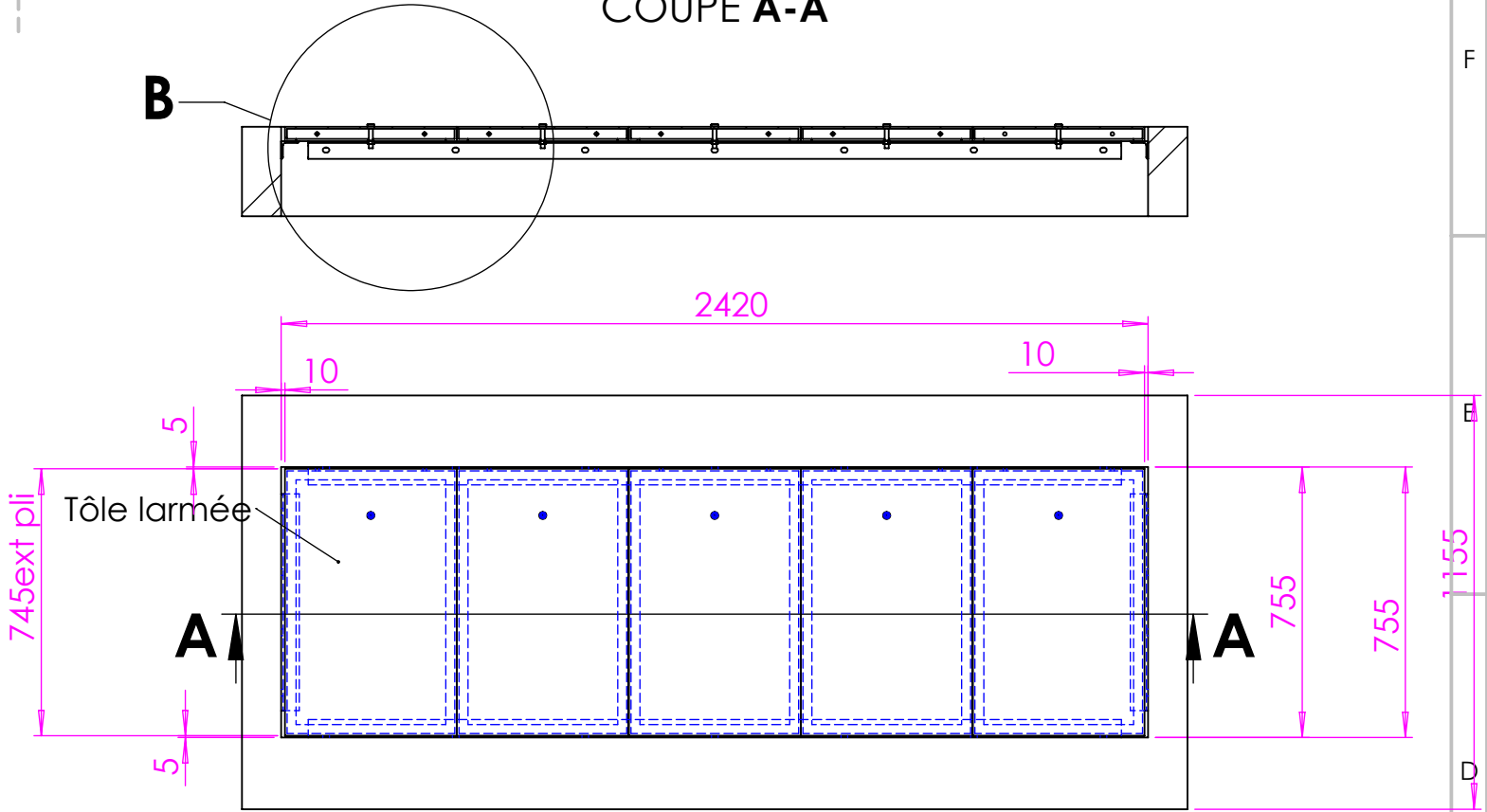
COUPE A-A
